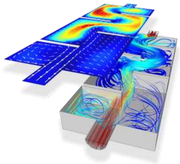
3D MODELY PROUDĚNÍ VZDUCHU
